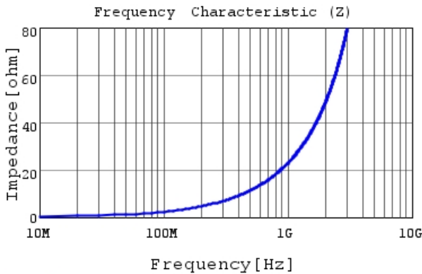
LQG15WH3N7S02 |Z|
