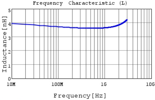
LQG15WH3N7S02 L
