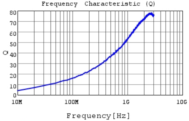
LQG15WH3N7S02 Q
