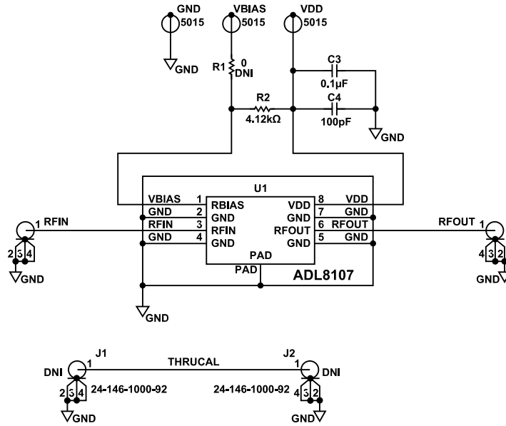
Figure 4. ADL8107-EVALZ Schematic
