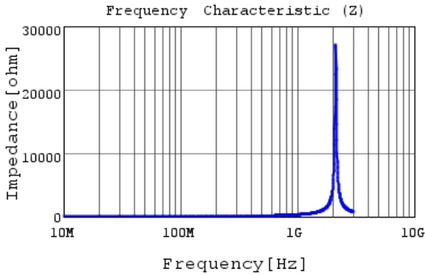
LQG15WH43NJ02 |Z|
