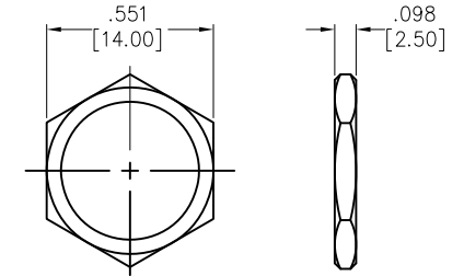
NUT
