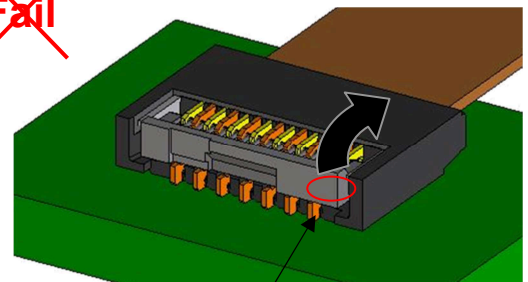
偏った部分での操作 Push up the one side of actuator
