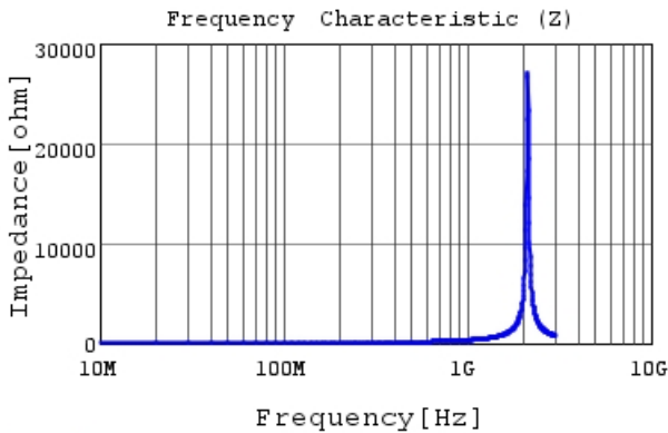
LQG15WH43NH02 |Z|
