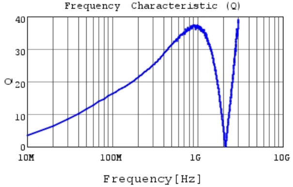
LQG15WH43NH02 Q
