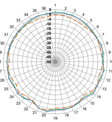
XZ-Plane Gain
