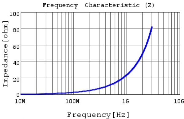
LQG15WH3N8S02 |Z|
