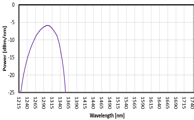
FIG. 7: SLED 6 SPECTRUM
