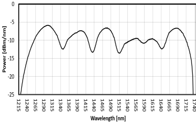
FIG. 1: ISB2 SPECTRUM
