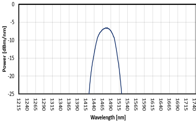
FIG. 7: SLED 6 SPECTRUM
