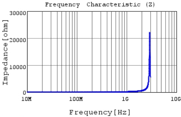
LQG15WZ24NG02 |Z|
