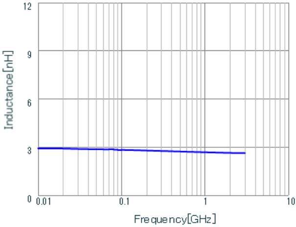
LQP02TQ2N7C02 L.
