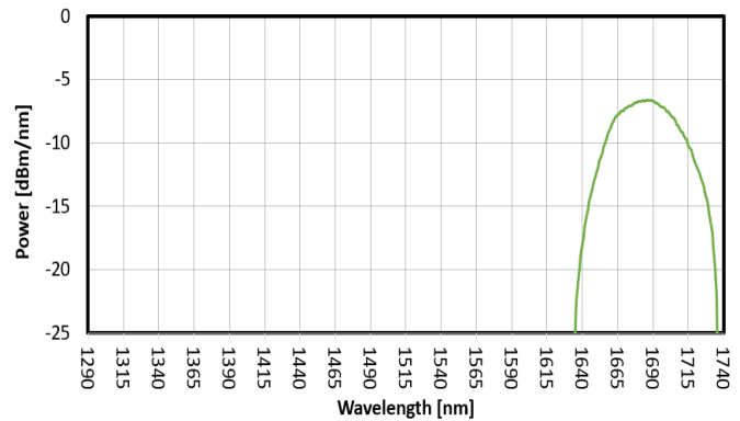
FIG. 2: SLED 1 SPECTRUM
