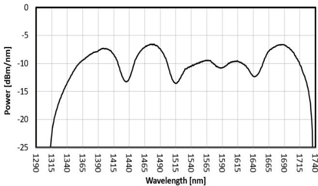
FIG. 1: OSE2 SPECTRUM
