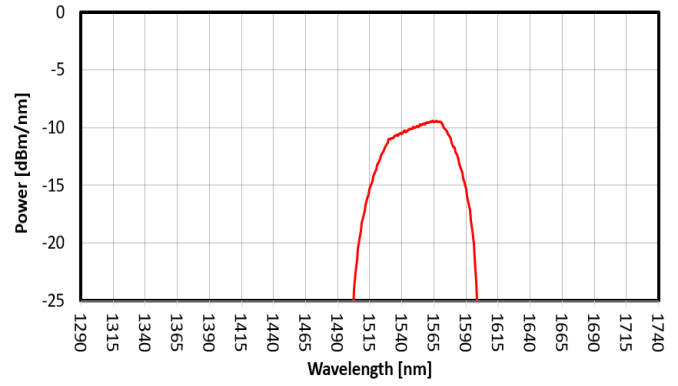
FIG. 4: SLED 3 SPECTRUM
