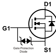
Q1 N-Channel
