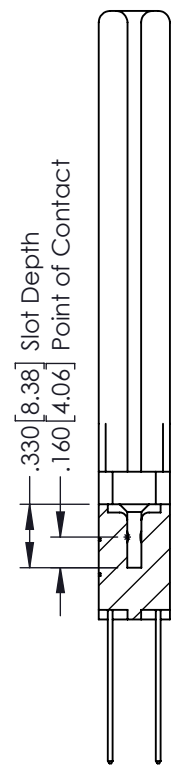
SECTION A-A
