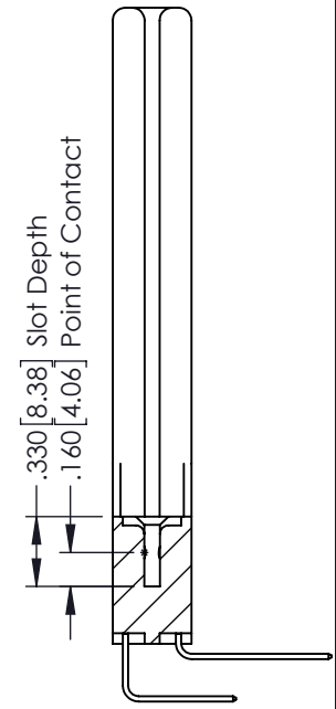
SECTION A-A
