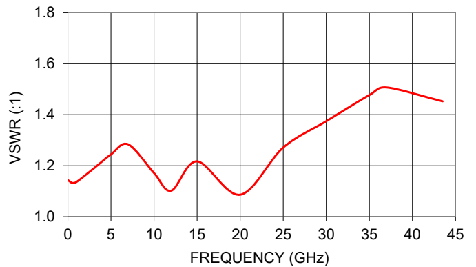
KAT-15+ VSWR
