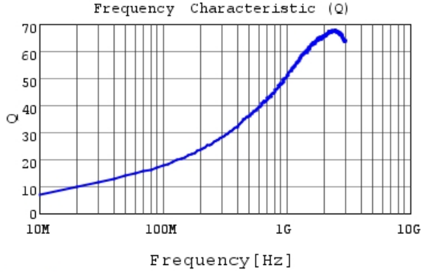
LQG15WH4N1B02 Q
