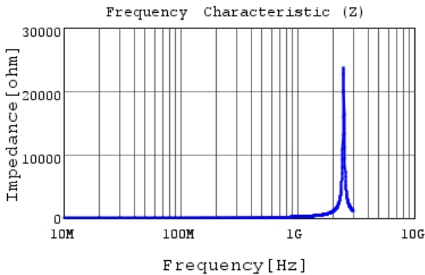
LQG15WH30NJ02 |Z|
