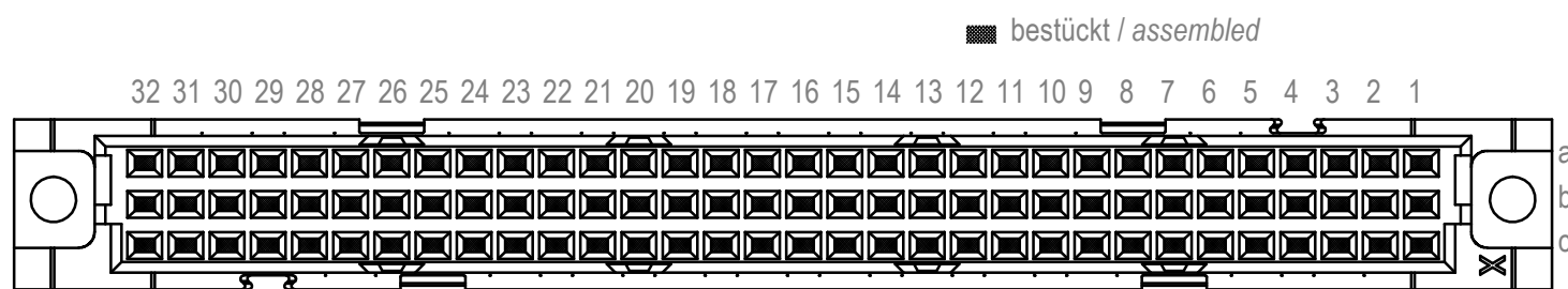
Bestückungsplan / contact layout
