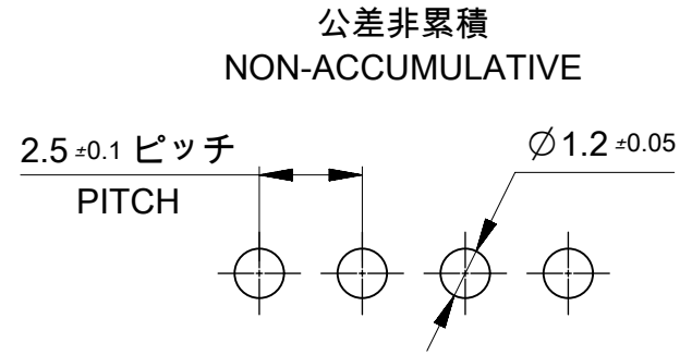
公差非累積 NON-ACCUMULATIVE 基板取付穴推奨寸法 RECOMMENDED P.C. BOARD HOLE DIM.
