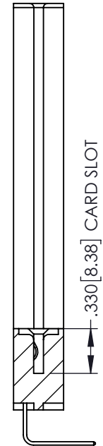
SECTION A-A
