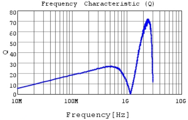
LQG15WHR12H02 Q
