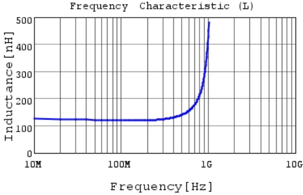
LQG15WHR12H02 L
