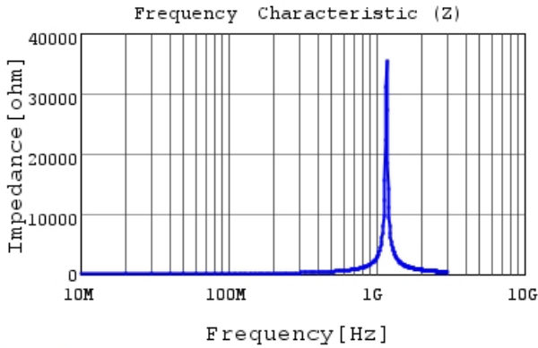
LQG15WHR12H02 |Z|
