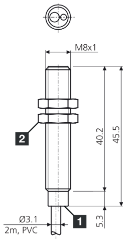
1) LED 2) Schlüsselweite 13 mm BK: schwarz BN: braun BU: blau
