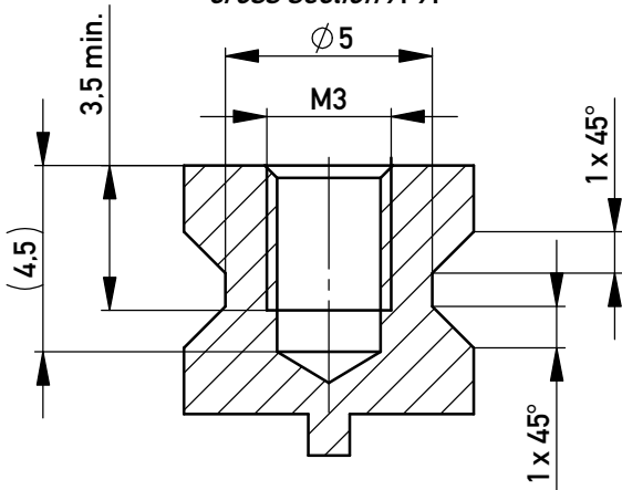
Schnitt A-A / cross section A-A
