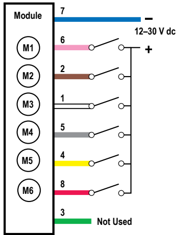
PNP Input
