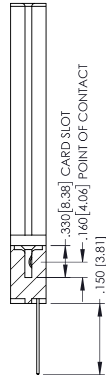
SECTION A-A
