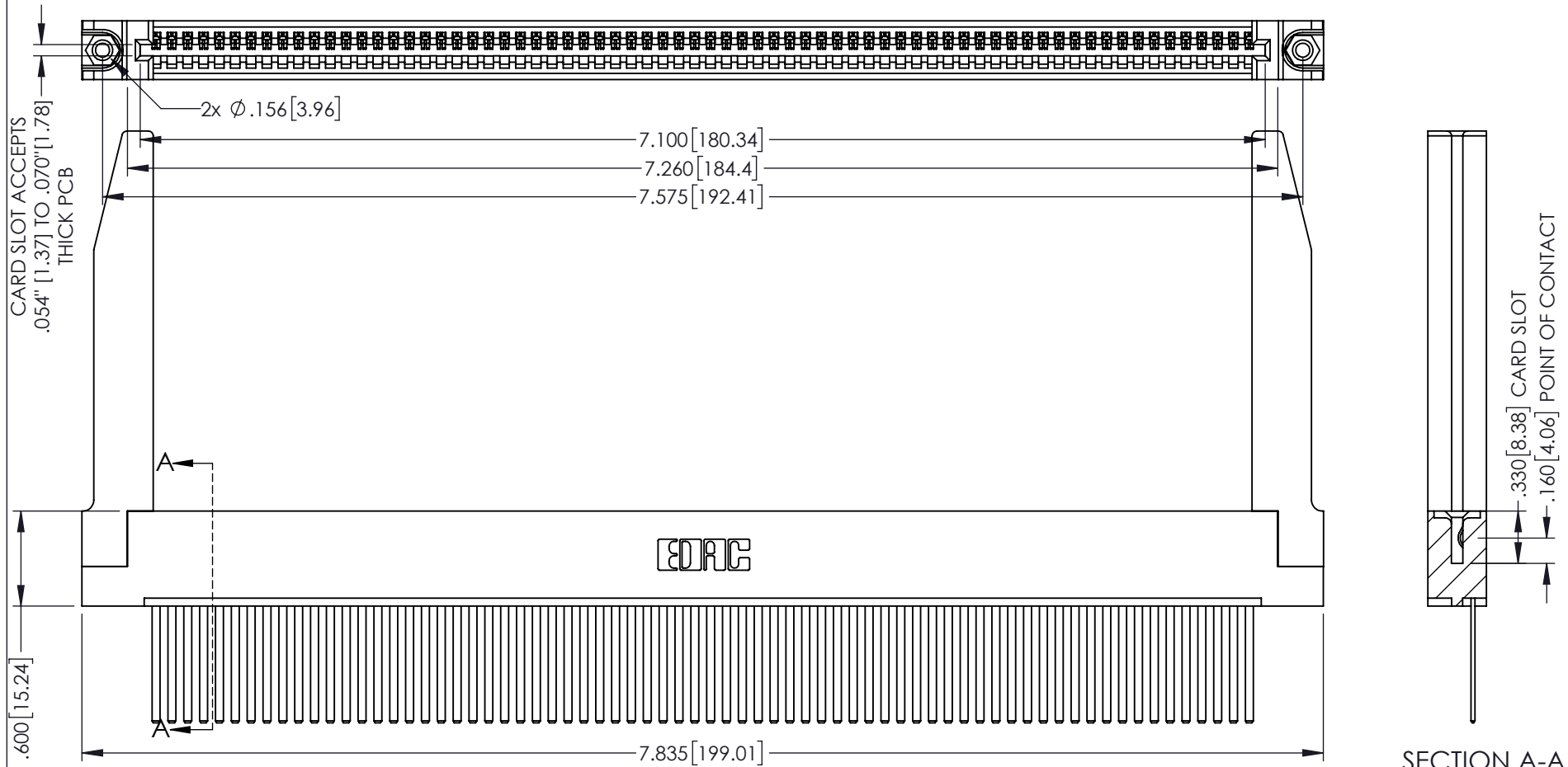
SECTION A-A
