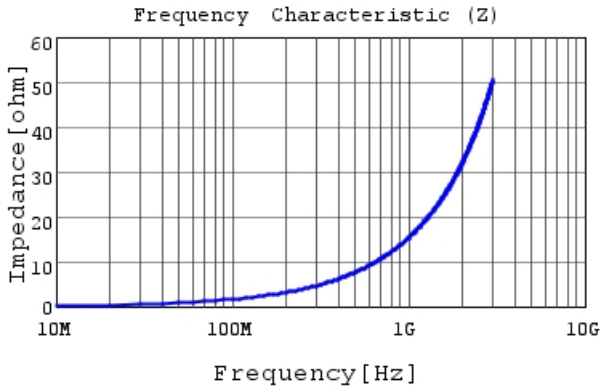
LQG15WH2N5B02 |Z|
