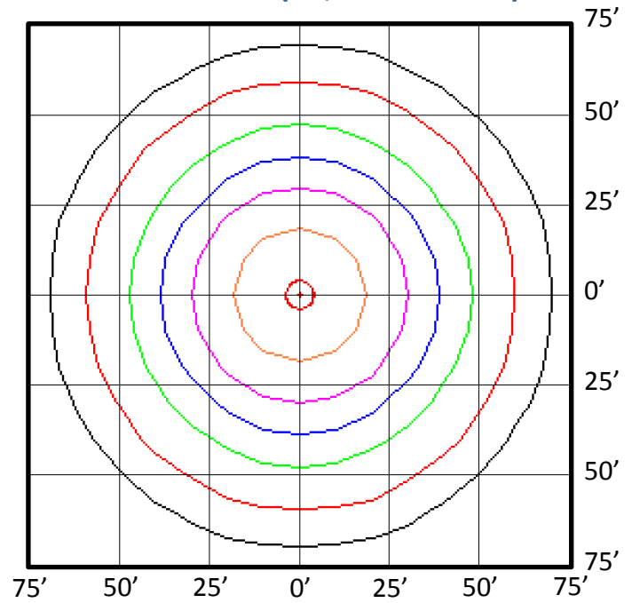
CLHB-RD-15050 (18,450 Lumens)
