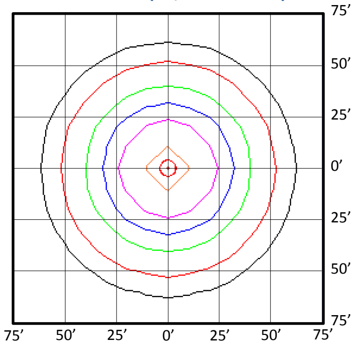
CLHB-RD-10050 (13,116 Lumens)
