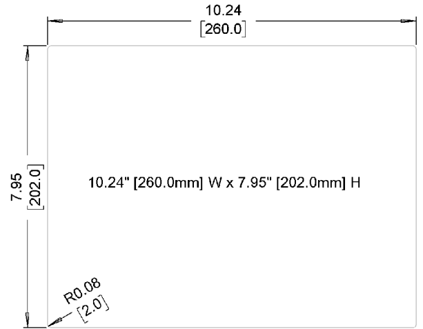
Cutout Dimensions
