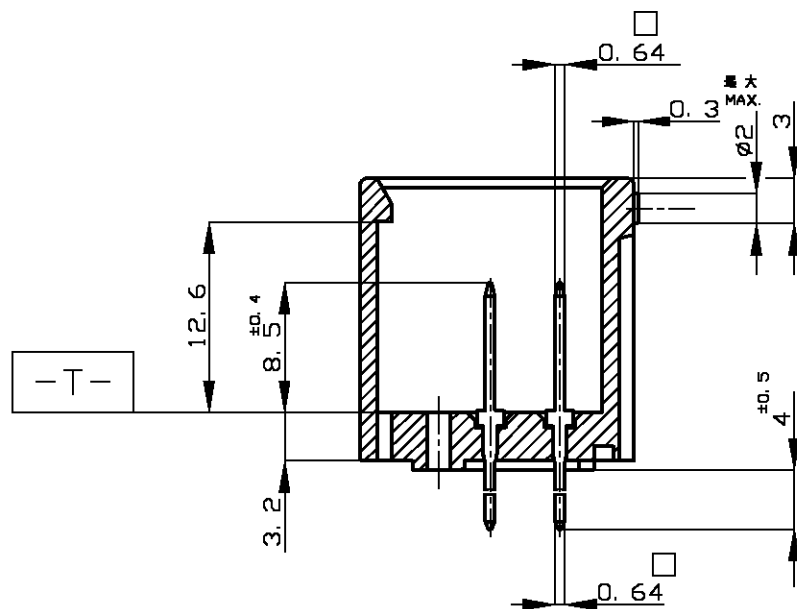
断面 A-A
