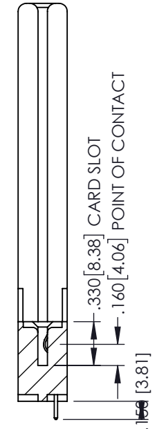
SECTION A-A
