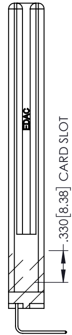
SECTION A-A
