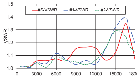
ZFRSC-183-S+ VSWR
