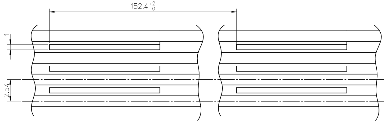
Numer narzedzia 158 - pojedyncze wyciecie Tool number 158 - single cut-out
