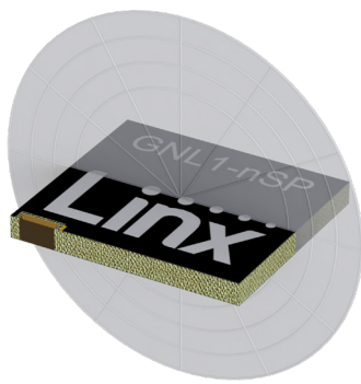
XZ-Plane Gain
