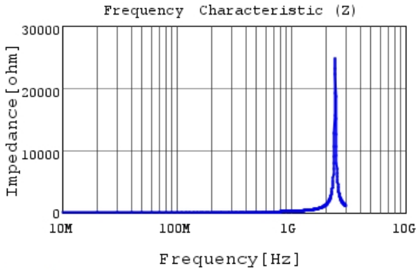
LQG15WZ33NH02 |Z|
