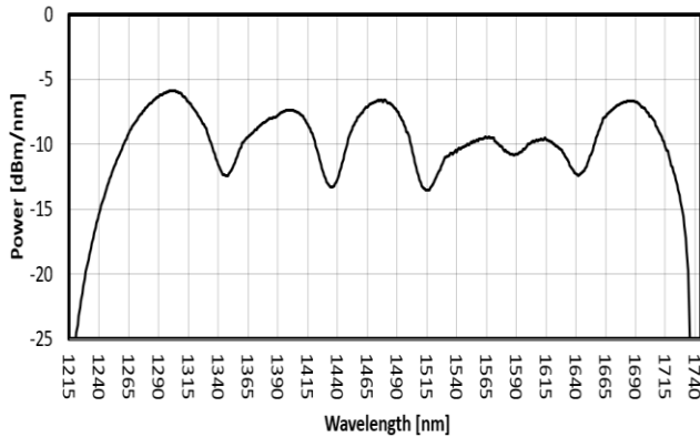
FIG. 1: ISB2 SPECTRUM
