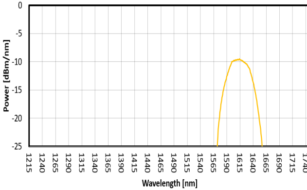
FIG. 3: SLED 2 SPECTRUM
