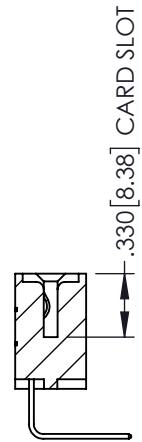
SECTION A-A
