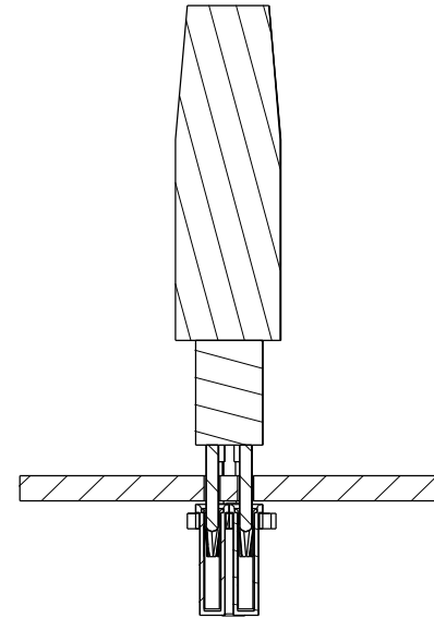
Section D-D
