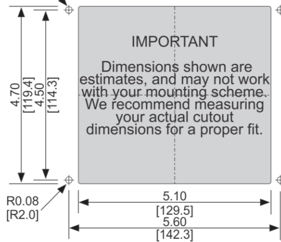
Cutout Dimensions
