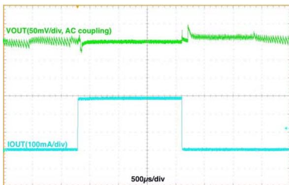
Figure 20. Load Transient, V_{IN} = 3.6\text{ V} , V_{OUT} = 1.8\text{ V} , 5\text{ mA} \Leftrightarrow 300\text{ mA} , 1\ \mu\text{s} Edge, Auto Mode
