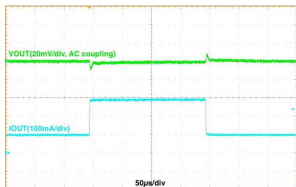
Figure 21. Load Transient, V_{IN} = 3.6\text{ V} , V_{OUT} = 1.8\text{ V} , 100\text{ mA} \Leftrightarrow 300\text{ mA} , 1\ \mu\text{s} Edge, Auto Mode
