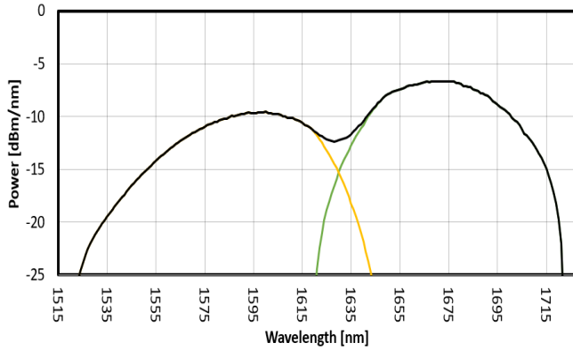
FIG. 1: OSE2 SPECTRUM
