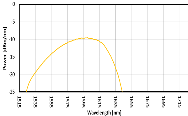
FIG. 3: SLED 2 SPECTRUM
