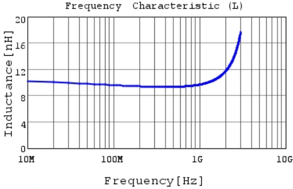
LQG15WH9N5H02 L
