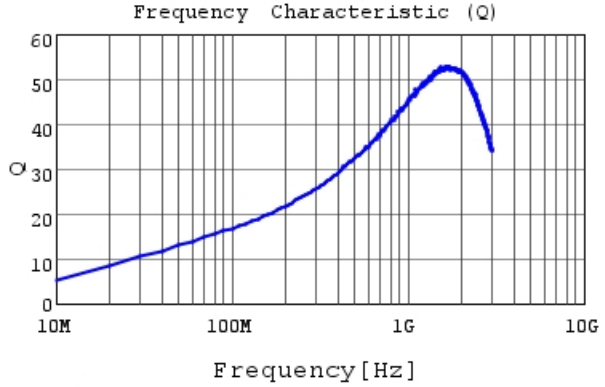
LQG15WH9N5H02 Q
