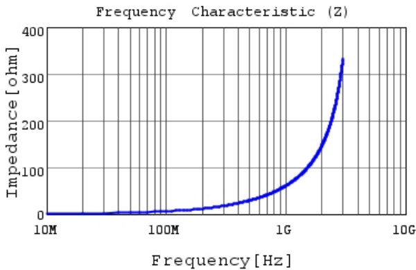
LQG15WH9N5H02 |Z|
