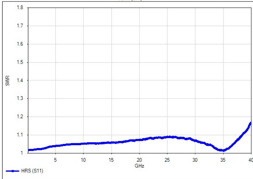
VSWR(S11)
